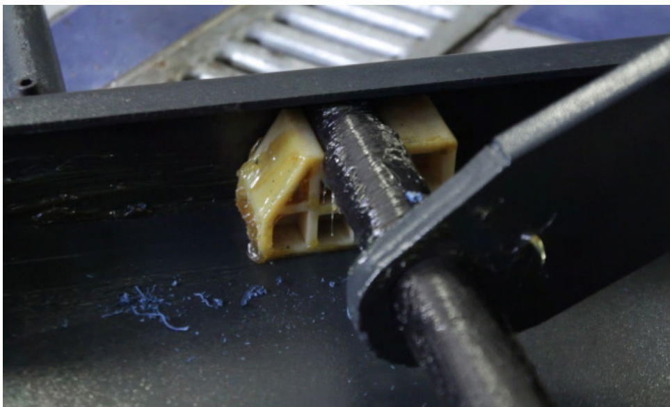
Auch diese Schiene muss geschmiert sein.
